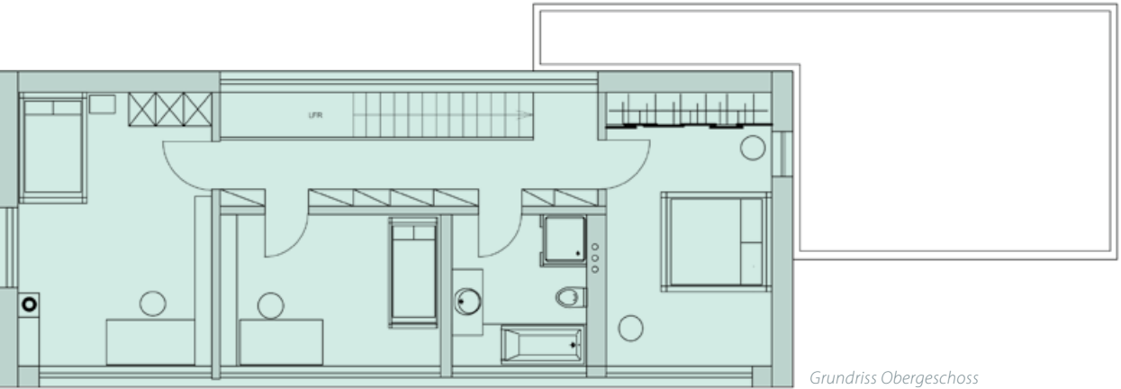
Grundriss Obergeschoss
