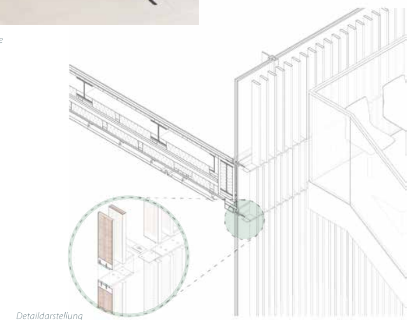
Detaildarstellung
